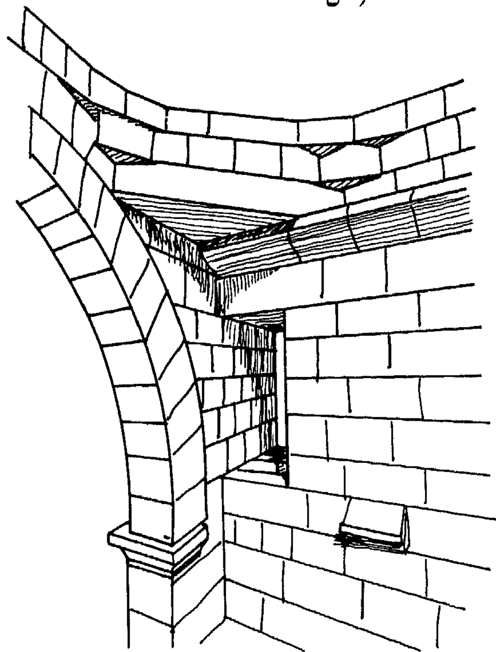
شكل (٢٣) وضع قبة مزار أم الزيتون (عن : Creswell, Fig.365)
